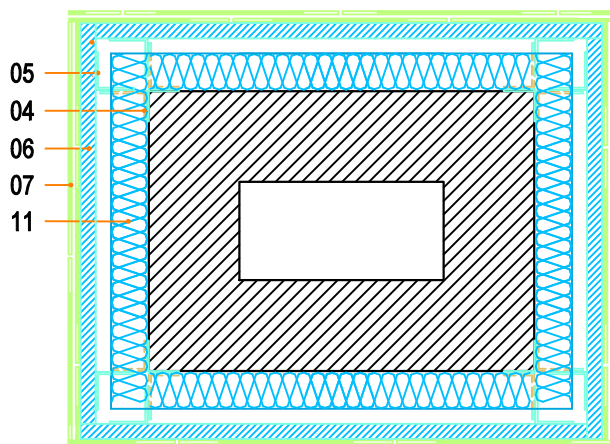
Pjūvis 1 – 1
